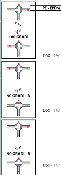
Válvulas de bola 3 vías PVC-U - 3 vías 3-way Series ball valves PVC-U - 3 ways
